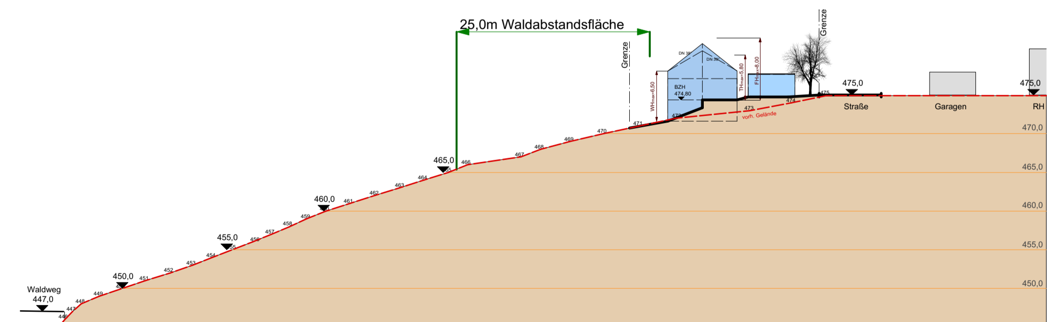
Schnitt E-F
