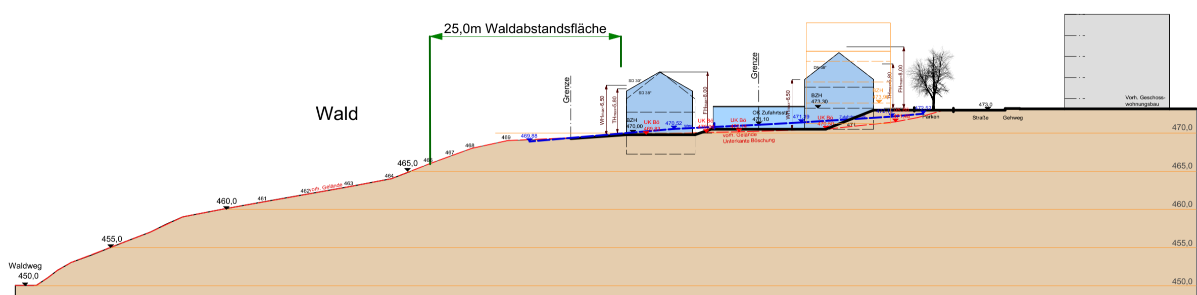
Schnitt C-D
