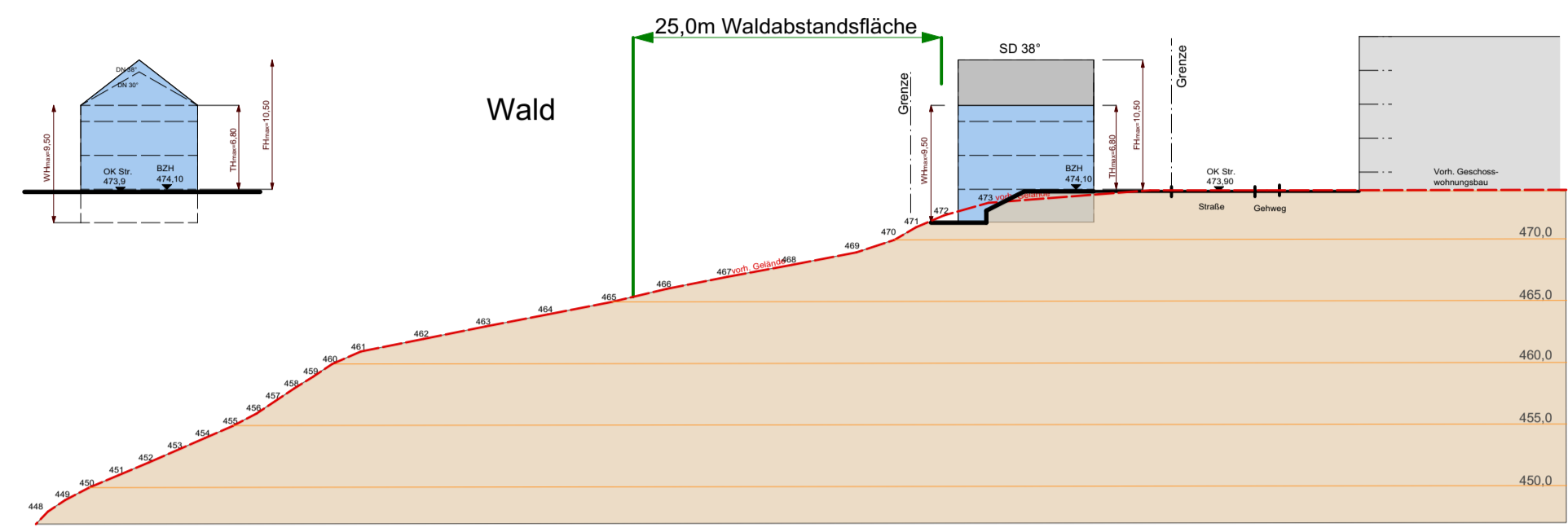
Schnitt A-B
